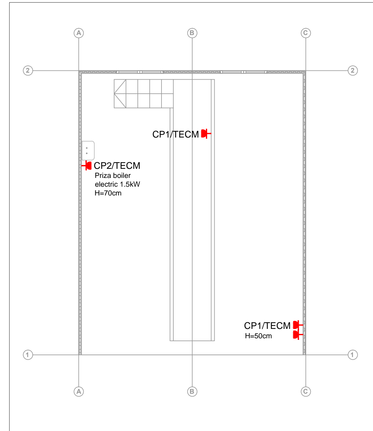
2. PLAN PRIZE CONTROL AMANUNTIT MICROBUZE SI MASINI MICI SCARA 1:50
