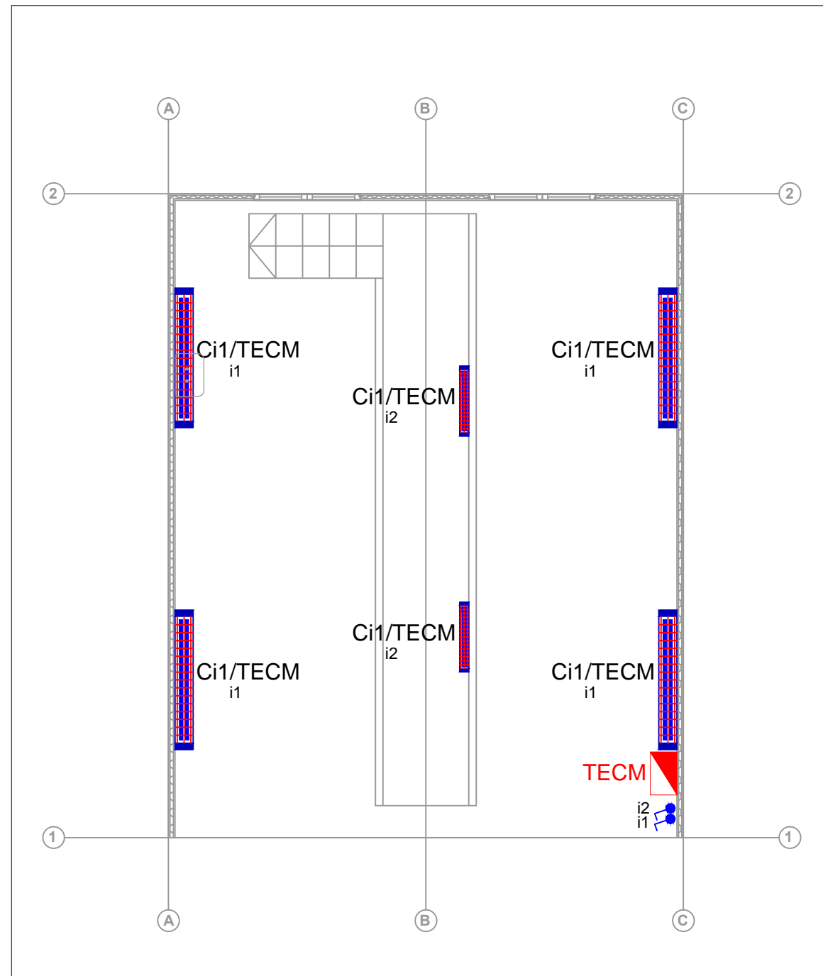
1. PLAN ILUMINAT CONTROL AMANUNTIT MICROBUZE SI MASINI MICI SCARA 1:50
